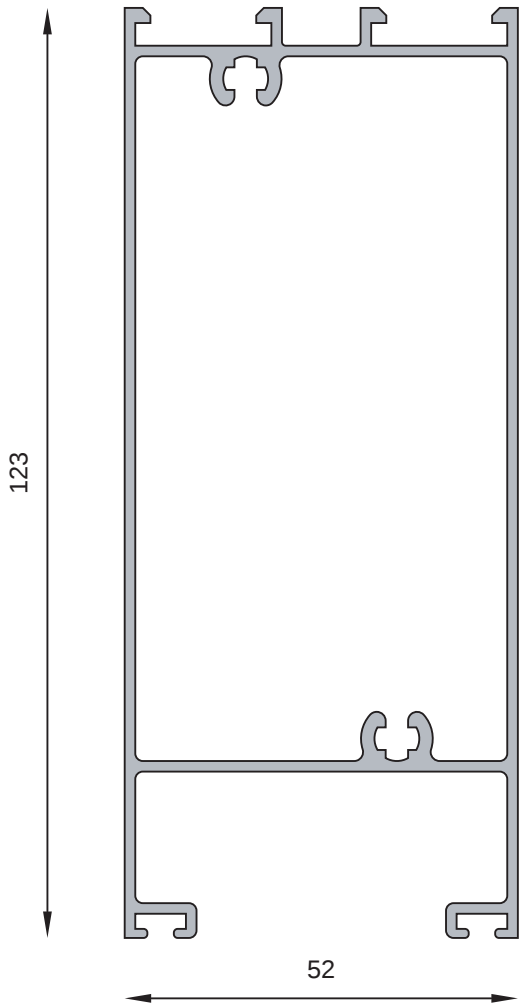
MT-0219 Zócalo hoja de puerta Peso estimado: 1.647 Kg/m
