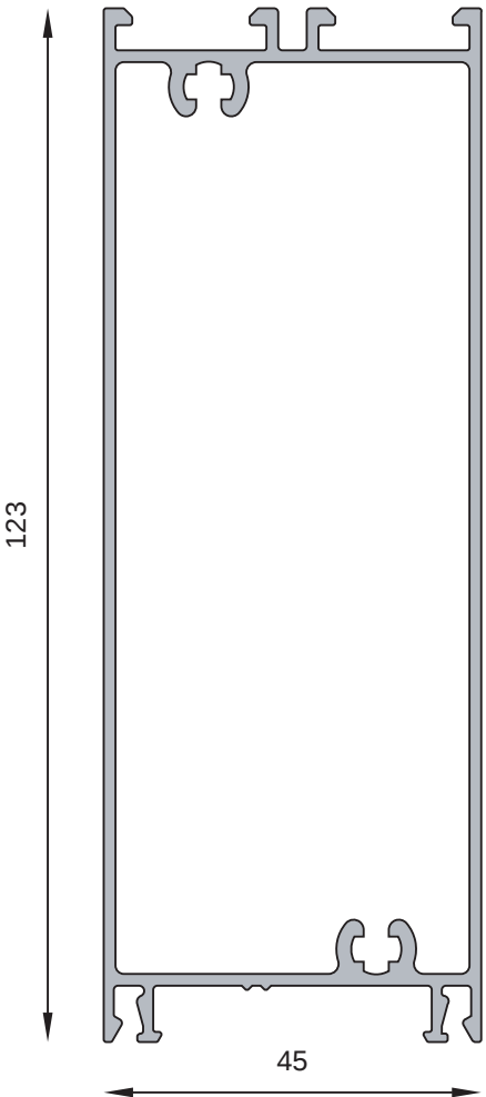
MT-0263 Zócalo alto paño fijo Peso estimado: 1.549 Kg/m
