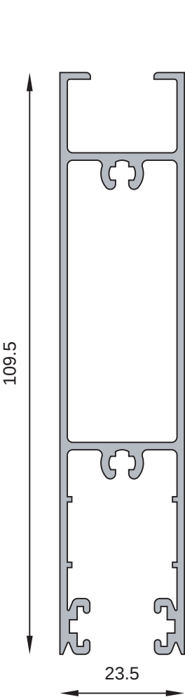
MT-0209 Zócalo alto Peso estimado: 1.255 Kg/m
