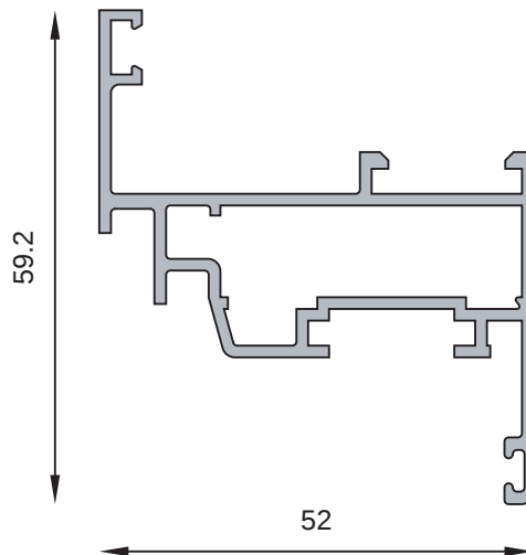
MT-0211 Hoja de abrir con cámara compensadora Peso estimado: 0.848 Kg/m
