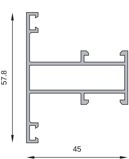
MT-0221 Travesaño angosto paño fijo Peso estimado: 0.767 Kg/m
