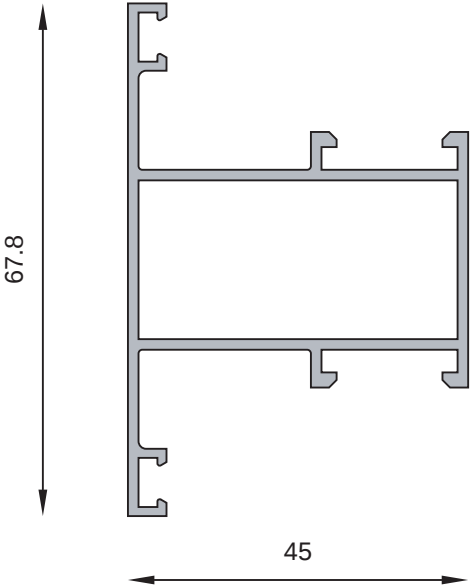
MT-0222 Travesaño ancho paño fijo Peso estimado: 0.839 Kg/m
