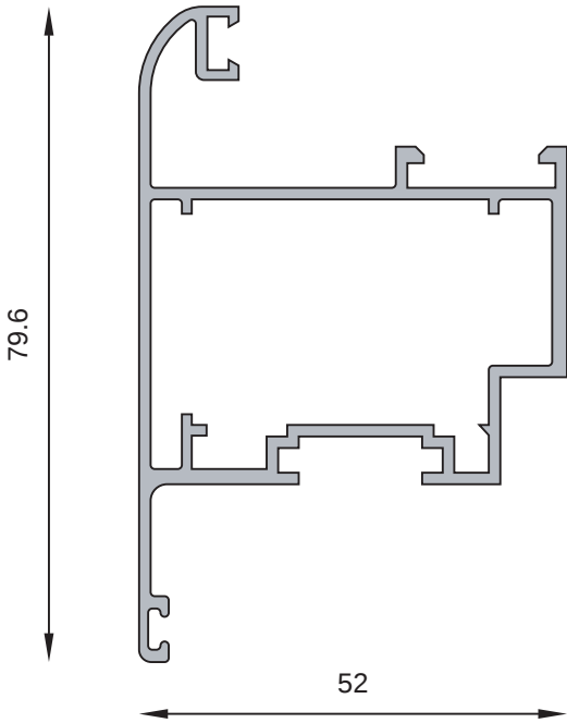
MT-0260 Hoja ventana proyectante curva Peso estimado: 1.099 Kg/m
