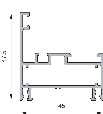
MT-0210 Marco de abrir con cámara compensadora Peso estimado: 0.785 Kg/m
