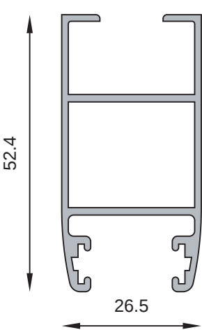
MT-0203 Parante Lateral Vidrio Simple Peso estimado: 0.661 Kg/m
