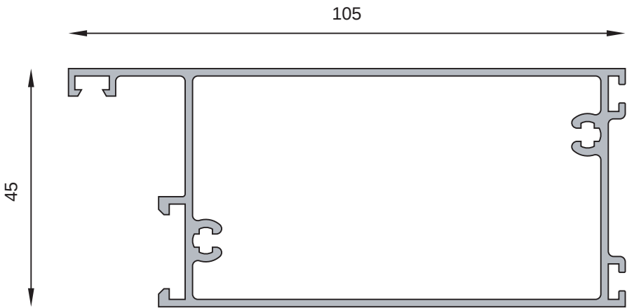
MT-0219 Zócalo hoja de puerta Peso estimado: 1.647 Kg/m
