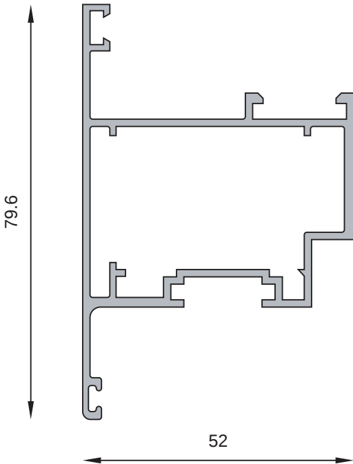
MT-0259 Marco ventana proyectante Peso estimado: 0.748 Kg/m
