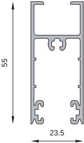
MT-0204 Zócalo y cabezal de hoja Peso estimado: 0.704 Kg/m
