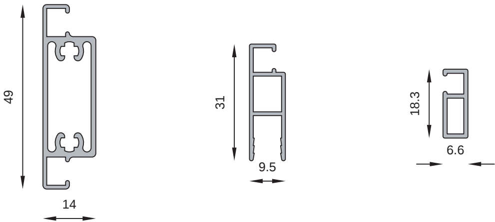
MT-0990 Travesaño de mosquitero Peso estimado: 0.486 Kg/m
