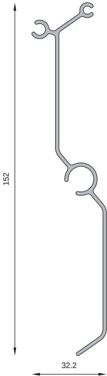
MT-2684 Tablilla parasol Peso estimado: 0.881 Kg/m
