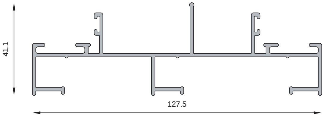
MT-0145 Marco doble de abrir Peso estimado: 1.325 Kg/m
