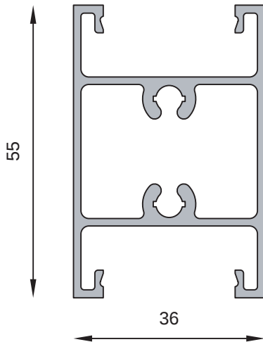
MT-2722 Travesaño celosía regulable Peso estimado: 0.992 Kg/m
