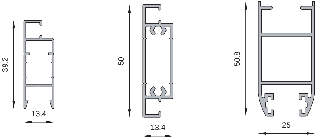
MT-1203 Hoja mosquitero Peso estimado: 0.265 Kg/m
