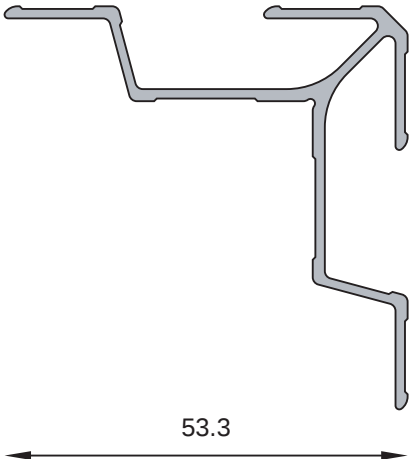
MT-0836 Escuadra universal liviana Peso estimado: 0.547 Kg/m
