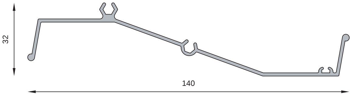
MT-0036 Tablilla parasol móvil Peso estimado: 0.772 Kg/m
