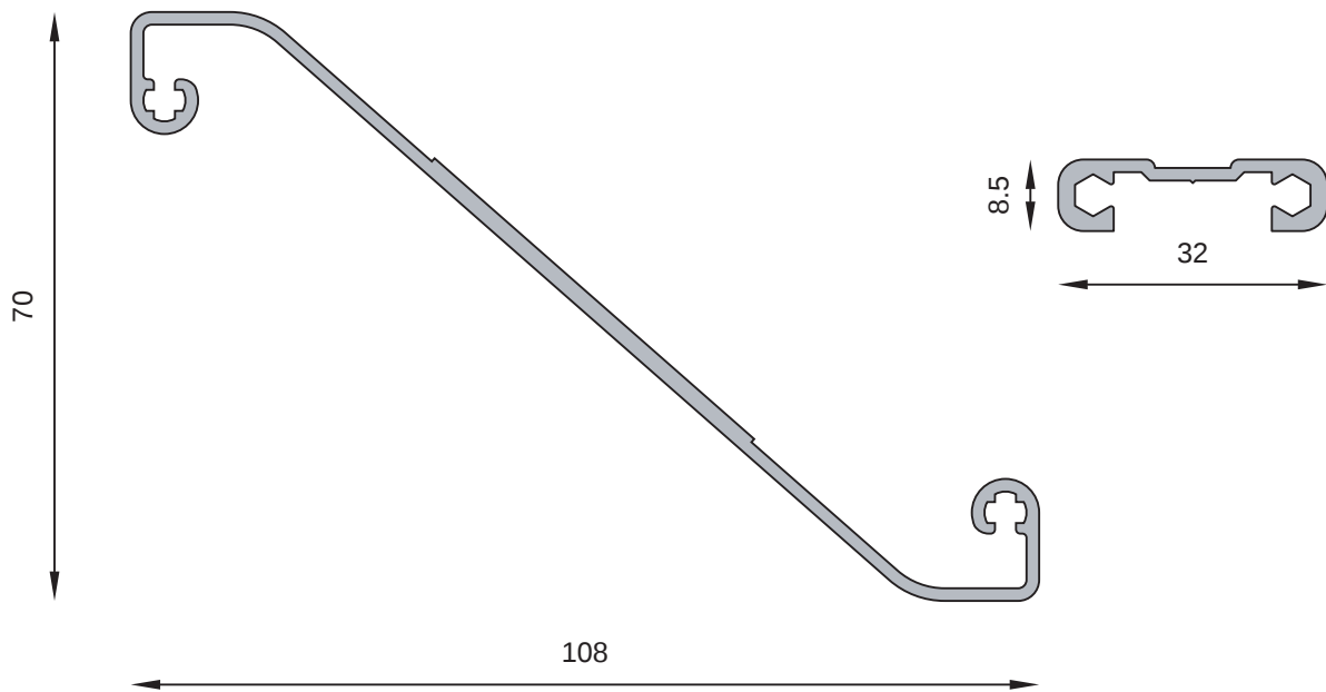
MT-0650 Parasol Peso estimado: 0.780 Kg/m
