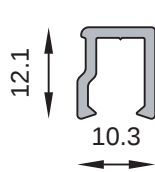
MT-0910 Contravidrio Peso estimado: 0.121 Kg/m
