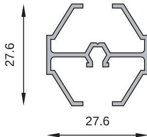
MT-2552 Travesaño universal vidrio repartido Peso estimado: 0.331 Kg/m
