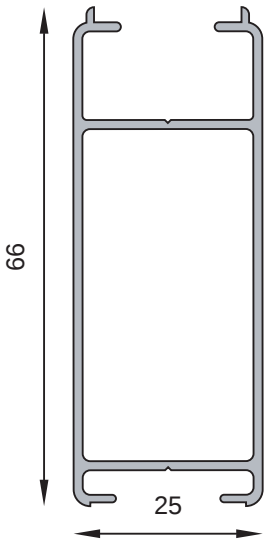
MT-0913 Batiente hoja rebatir 25 mm Peso estimado: 0.625 Kg/m
