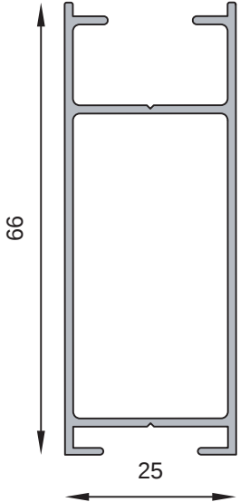
MT-2734 Batiente hoja Peso estimado: 0.634 Kg/m
