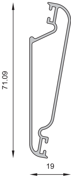
MT-2705 Tablilla celosía regulable Peso estimado: 0.532 Kg/m
