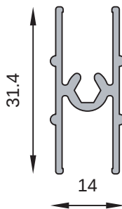
MT-1346 Travesaño intermedio hoja cubrebañera Peso estimado: 0.305 Kg/m
