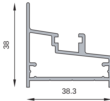
MT-0188 Marco cubre-duchador Peso estimado: 0.567 Kg/m
