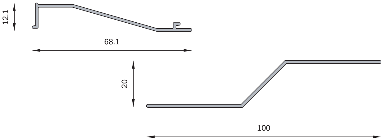
MT-0006 Tablilla postigón Peso estimado: 0.267 Kg/m
