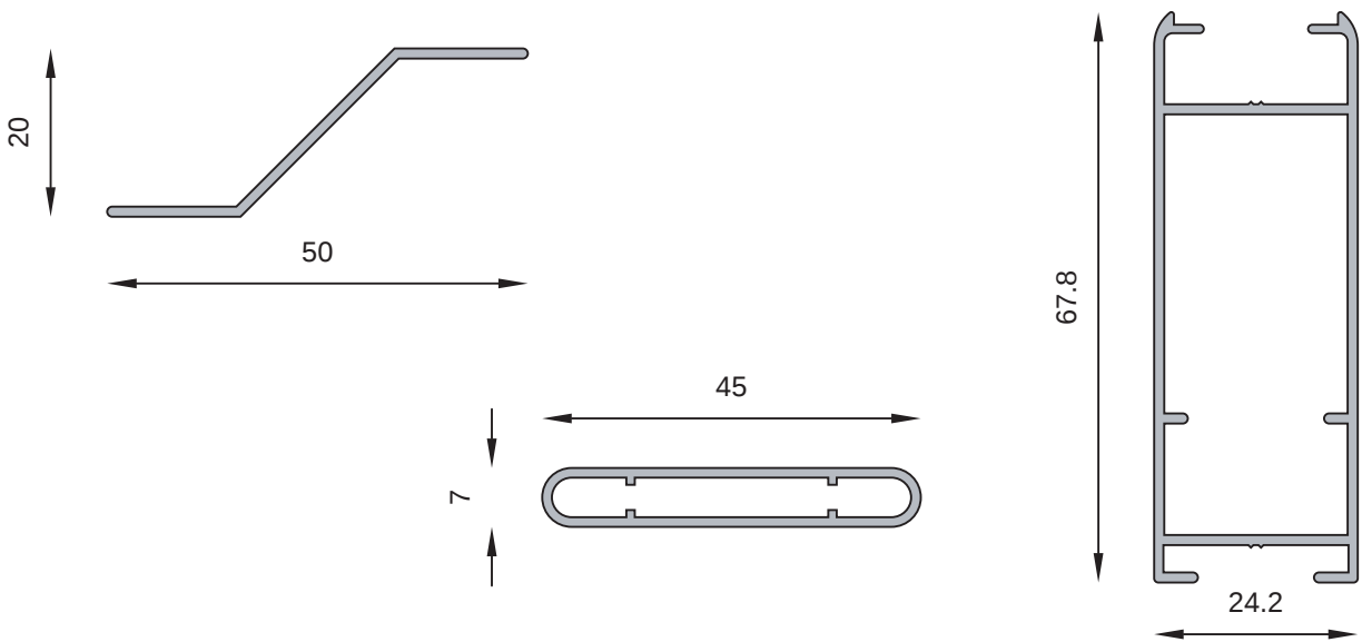
MT-0153 Tablilla fija para postigón Peso estimado: 0.186 Kg/m
