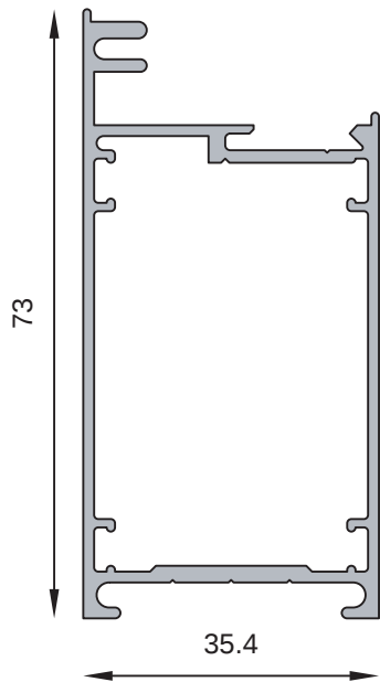
MT-2850 Marco perimetral de hoja puerta 35 mm Peso estimado: 0.913 Kg/m
