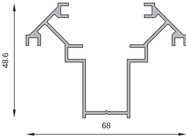
MT-1391 Columna tabique divisorio Peso estimado: 0.729 Kg/m
