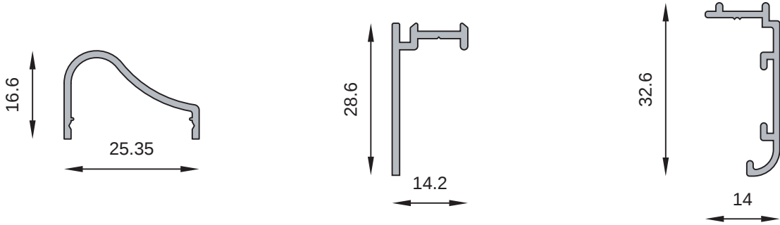
MT-2692 Moldura puerta placa Peso estimado: 0.163 Kg/m
