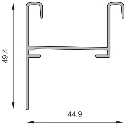
MT-0945 Marco dos guías con tapajunta para corredizas Peso estimado: 0.465 Kg/m
