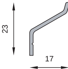
MT-1913 Botagua Peso estimado: 0.126 Kg/m
