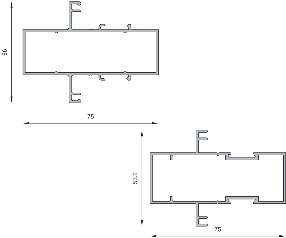
MT-0994 Travesaño paño fijo Peso estimado: 0.928 Kg/m
