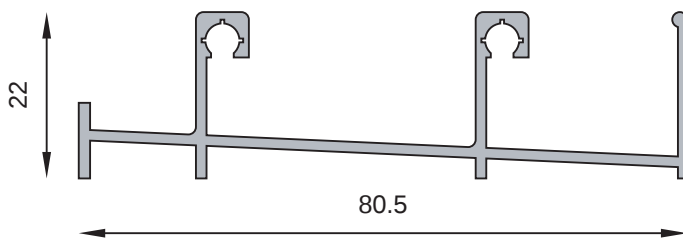
MT-1318 Guía con tope para corrediza Peso estimado: 0.660 Kg/m
