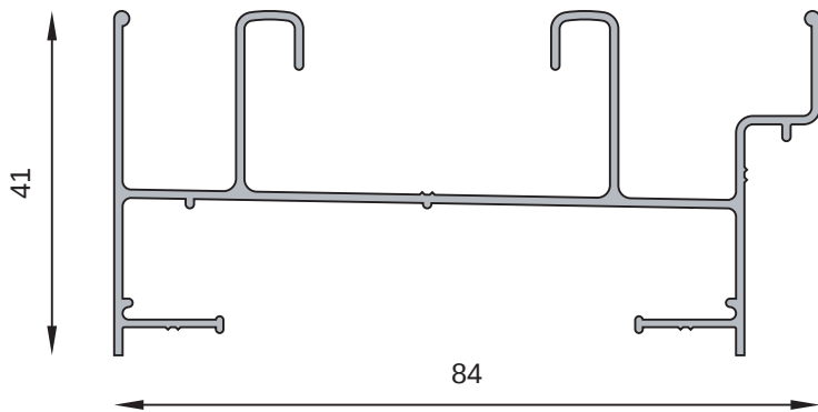
MT-0901 Marco perimetral Peso estimado: 0.713 Kg/m
