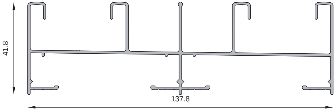
MT-0714 Marco de cuatro guías para hojas corredizas Peso estimado: 1.314 Kg/m
