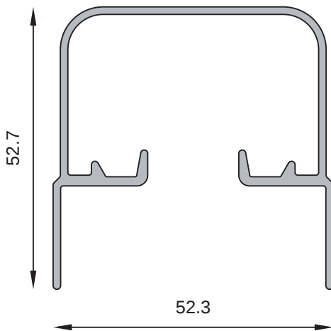
MT-1345 Cabezal cubrebañera Peso estimado: 0.774 Kg/m
