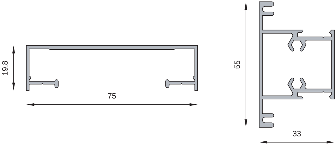
MT-0024 Marco puerta vai-ven Peso estimado: 0.577 Kg/m
