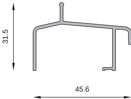
MT-0169 Umbral cubrebañera Peso estimado: 0.386 Kg/m
