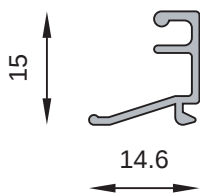
MT-0806 Contravidrio Peso estimado: 0.113 Kg/m
