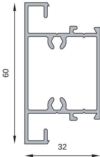
MT-2473 Travesaño ancho "Ibiza" Peso estimado: 0.744 Kg/m
