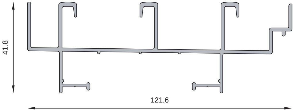
MT-0691 Marco de tres guías para hojas corredizas Peso estimado: 1.320 Kg/m
