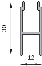
MT-1012 Umbral vitrina Peso estimado: 0.241 Kg/m
