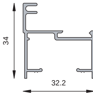
MT-0973 Paño fijo Peso estimado: 0.360 Kg/m
