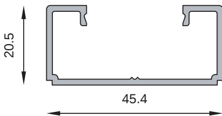
MT-2765 Adaptador celosía regulable en puerta 44 mm Peso estimado: 0.437 Kg/m
