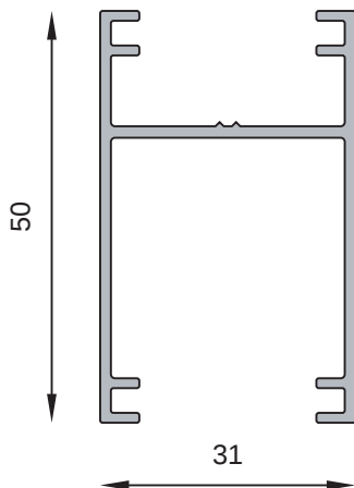
MT-0892 Travesaño Peso estimado: 0.549 Kg/m
