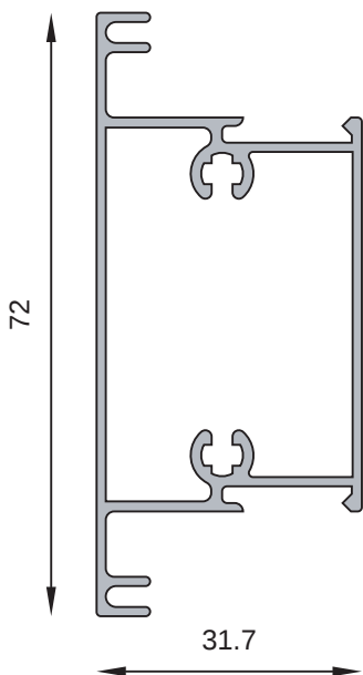
MT-0933 Travesaño hoja Peso estimado: 0.749 Kg/m
