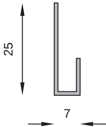
MT-1003 Perfil J 7 x 25 mm Peso estimado: 0.108 Kg/m
