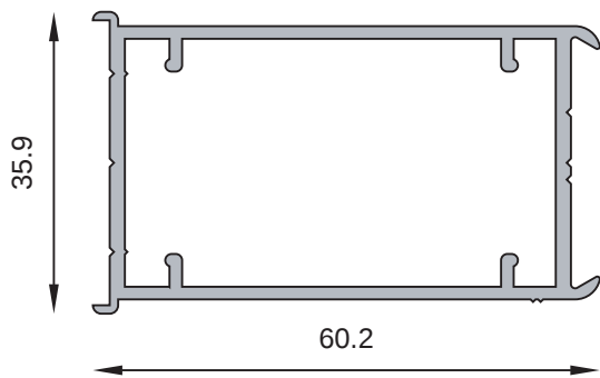
MT-0509 Hoja puerta de rebatir Peso estimado: 0.840 Kg/m
