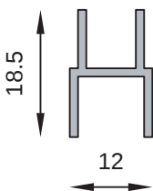
MT-2708 Calce tapaluz celosía regulable Peso estimado: 0.151 Kg/m
