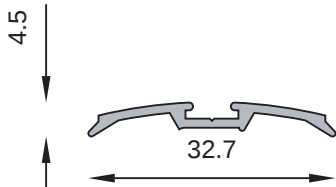
MT-0011 Travesaño puerta de rebatir Peso estimado: 1.713 Kg/m
