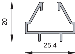
MT-0972 Perimetral vidrio repartido Peso estimado: 0.223 Kg/m
