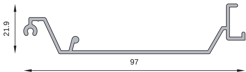
MT-0129 Tapa cinta Peso estimado: 0.587 Kg/m
