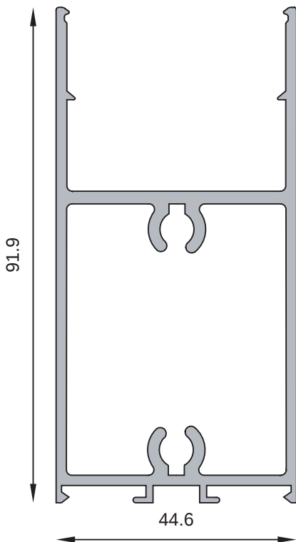
MT-0011 Travesaño puerta de rebatir Peso estimado: 1.713 Kg/m
