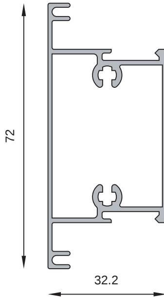
MT-0959 Travesaño intermedio puerta de rebatir Peso estimado: 0.799 Kg/m
