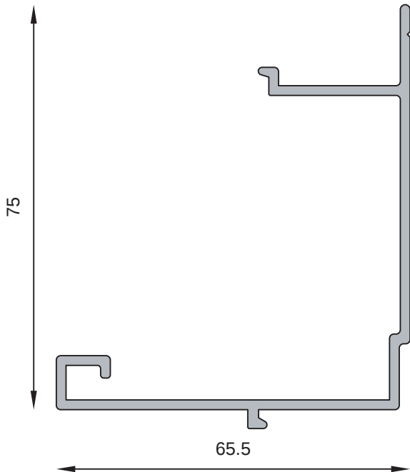
MT-2924 Guía techo corredizo Peso estimado: 0.933 Kg/m
