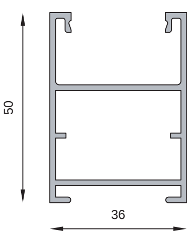
MT-2693 Hoja celosía regulable Peso estimado: 0.787 Kg/m
