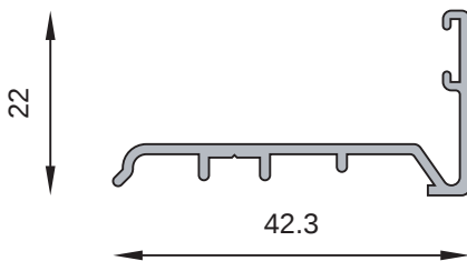
MT-0814 Tapacanto central Peso estimado: 0.240 Kg/m
