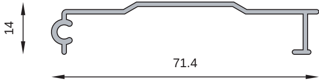
MT-1214 Tapa cinta Peso estimado: 0.334 Kg/m
