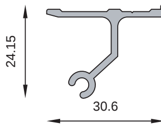
MT-0915 Bisagra ventana proyectante o banderola Peso estimado: 0.279 Kg/m
