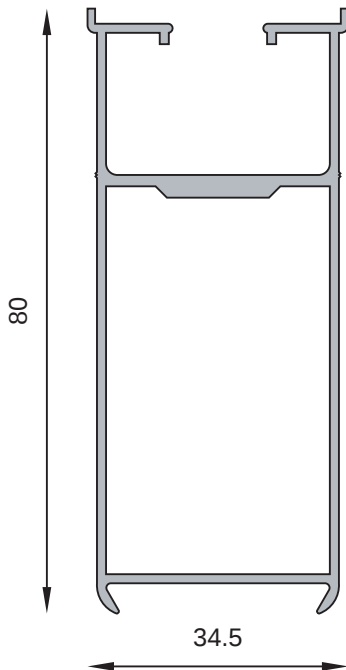
MT-2474 Hoja ventana "Ibiza" Peso estimado: 0.651 Kg/m
