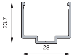
MT-0919 Adaptador para DVH en hojas corredizas Peso estimado: 0.272 Kg/m
