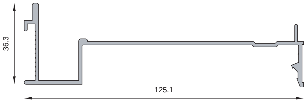
MT-0837 Escuadra universal Peso estimado: 0.725 Kg/m
