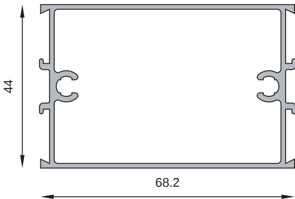
MT-0842 Travesaño puerta Peso estimado: 0.949 Kg/m
