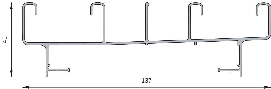
MT-0969 Marco unificado cuatro guías para hojas corredizas Peso estimado: 0.168 Kg/m
