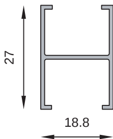
MT-2773 Travesaño vidrio repartido Peso estimado: 0.213 Kg/m
