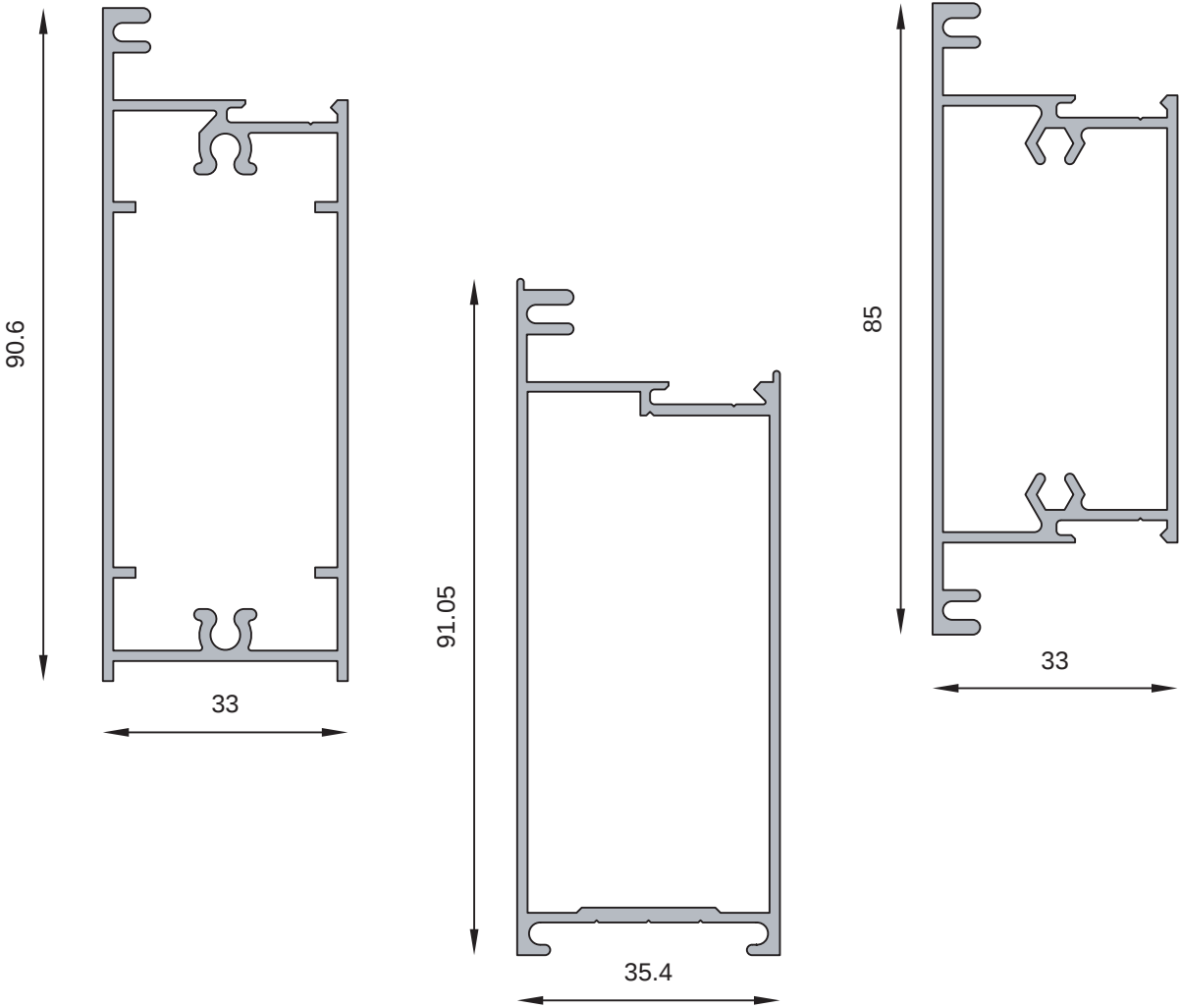
MT-2845 Travesaño inferior puerta 33 mm Peso estimado: 1.110 Kg/m
