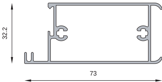
MT-1191 Puerta 33 mm, Zocalo y cabezal de hoja Peso estimado: 0.845 Kg/m
