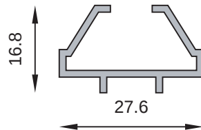
MT-2553 Marco universal vidrio repartido Peso estimado: 0.239 Kg/m
