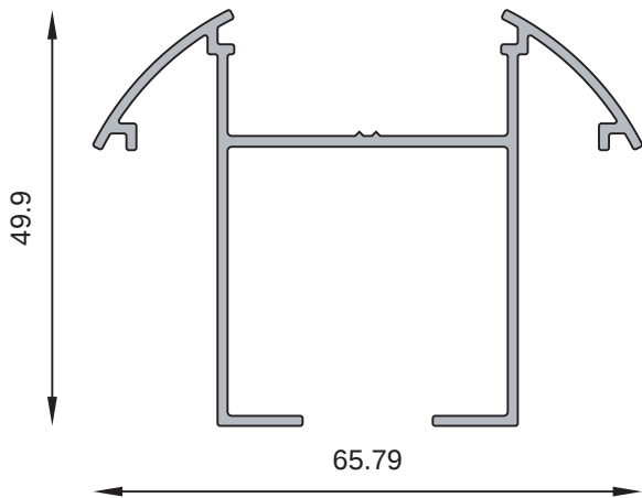
MT-0890 Columna Peso estimado: 0.678 Kg/m
