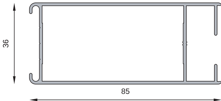
MT-0839 Parante puerta Peso estimado: 0.913 Kg/m
