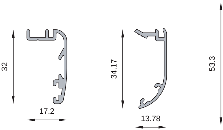
MT-0954 Premarco Peso estimado: 0.696 Kg/m
