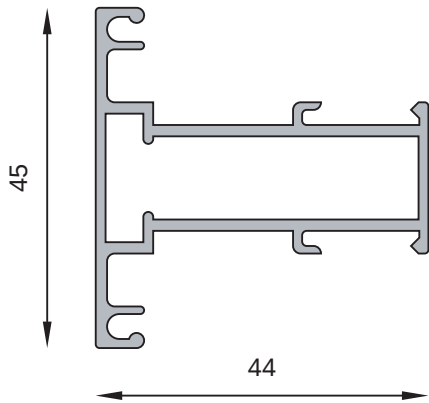
MT-0809 Travesaño repartido Peso estimado: 0.713 Kg/m
