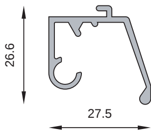
MT-0128 Soporte Tapa cinta Peso estimado: 0.339 Kg/m
