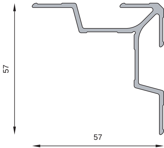
MT-0837 Escuadra universal Peso estimado: 0.725 Kg/m
