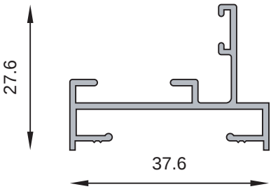
MT-0846 Marco de postigón para puerta Peso estimado: 0.335 Kg/m
