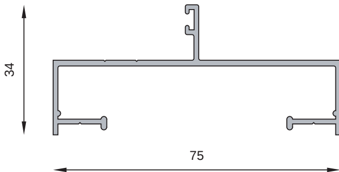
MT-0681 Marco puerta de rebatir Peso estimado: 0.599 Kg/m
