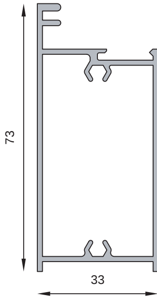
MT-2851 Travesaño superior puerta 33 mm Peso estimado: 0.872 Kg/m
