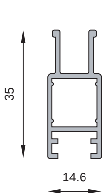
MT-0169 Umbral cubrebañera Peso estimado: 0.386 Kg/m
