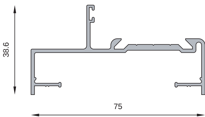
MT-0811 Marco de puerta encolizada Peso estimado: 0.761 Kg/m
