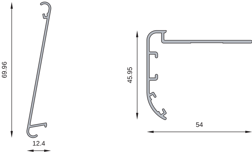
MT-0996 Tablilla Peso estimado: 0.265 Kg/m
