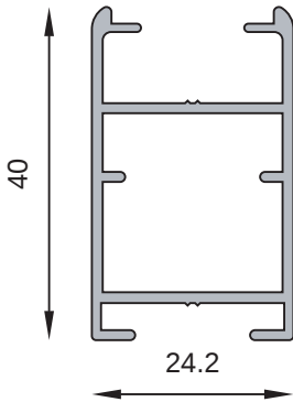
MT-0963 Hoja postigón Peso estimado: 0.495 Kg/m
