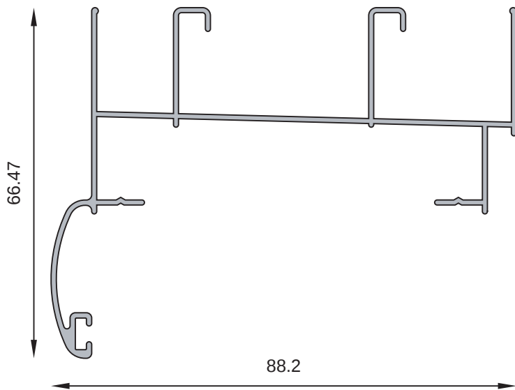
MT-1004 Marco con solapa Peso estimado: 0.748 Kg/m
