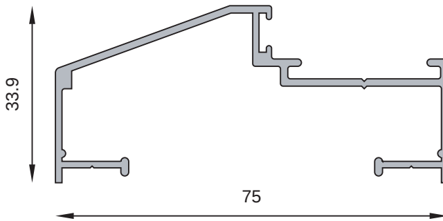
MT-2475 Hoja ventana "Ibiza" Peso estimado: 0.781 Kg/m
