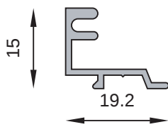
MT-0078 Contravidrio Peso estimado: 0.151 Kg/m
