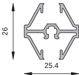
MT-0971 Travesaño vidrio repartido Peso estimado: 0.348 Kg/m
