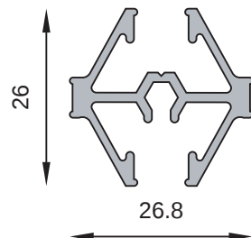
MT-2425 Travesaño vidrio repartido Peso estimado: 0.414 Kg/m
