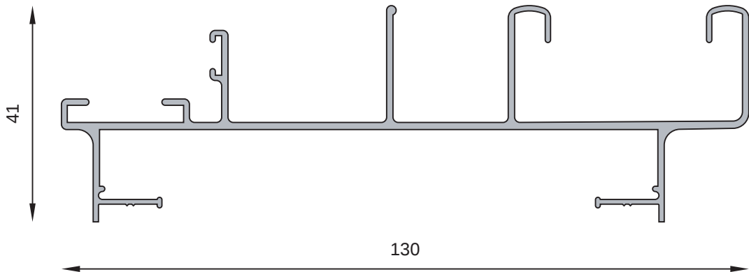
MT-0965 Marco unificado postigón corrediza Peso estimado: 1.069 Kg/m
