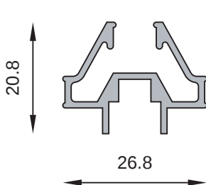
MT-2426 Perimetral vidrio repartido Peso estimado: 0.316 Kg/m
