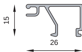
MT-0805 Contravidrio Peso estimado: 0.192 Kg/m
