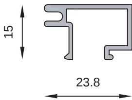
MT-0077 Contravidrio Peso estimado: 0.222 Kg/m
