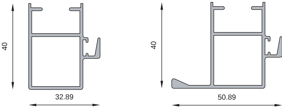
MT-2718 Parante central hoja corrediza "Monaco" Peso estimado: 0.578 Kg/m
