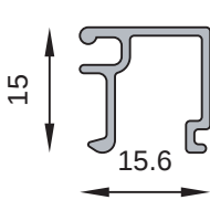
MT-0908 Contravidrio universal Peso estimado: 0.148 Kg/m
