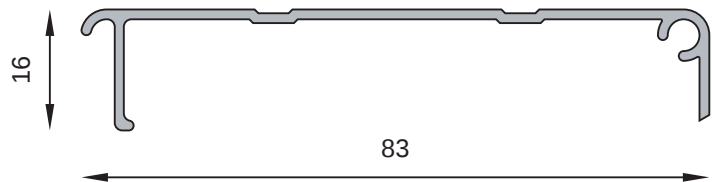
MT-0921 Tapa cinta Peso estimado: 0.414 Kg/m
