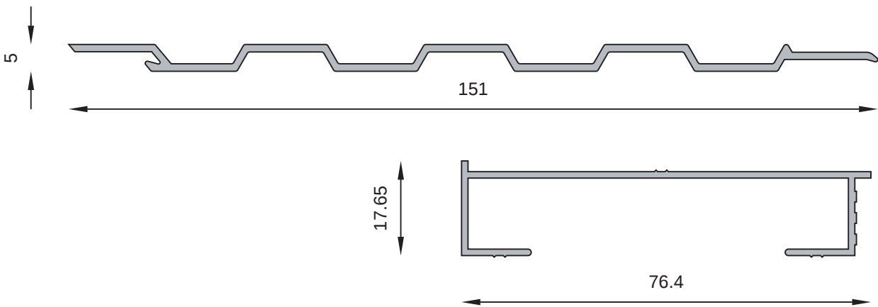
MT-0992 Revestimiento doble faz Peso estimado: 0.636 Kg/m
