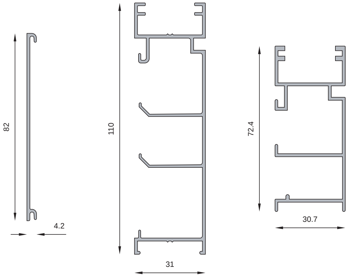
MT-0898 Tapa zócalo Peso estimado: 0.320 Kg/m
