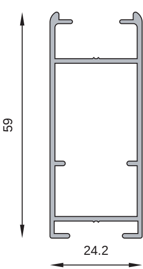
MT-0952 Parante hoja recto Peso estimado: 0.622 Kg/m
